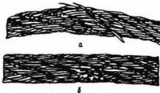
Рис. 3. Обрывы проволок в зоне уравнительного блока: а - в нескольких прядях каната; б - в двух прядях в сочетании с местным износом
